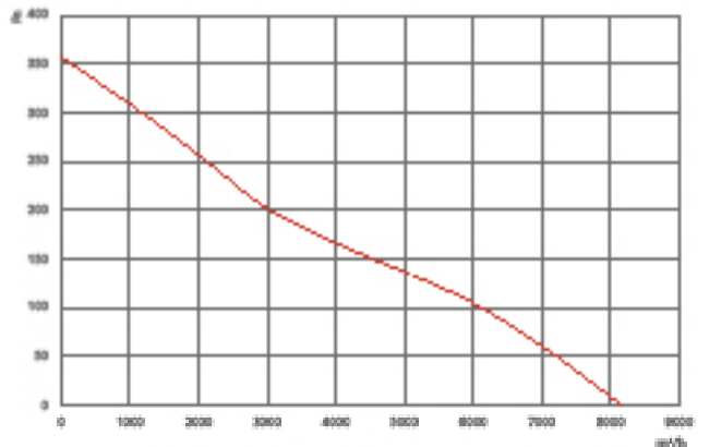
NFDAX/BX 560-5-25
