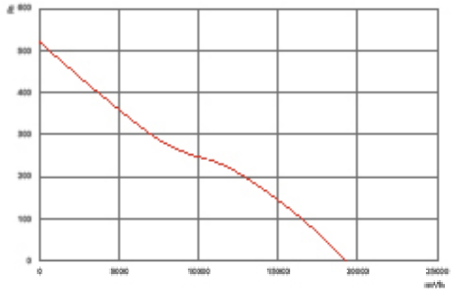
NFDAX/BX 710-5-30
