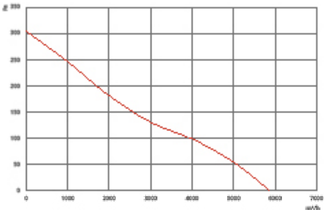
NFDAX/BX 500-5-25
