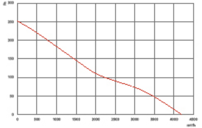
NFDAX/BX 450-5-25
