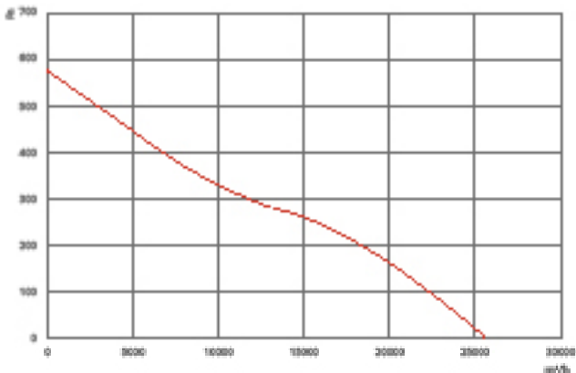
NFDAX/BX 800-5-30
