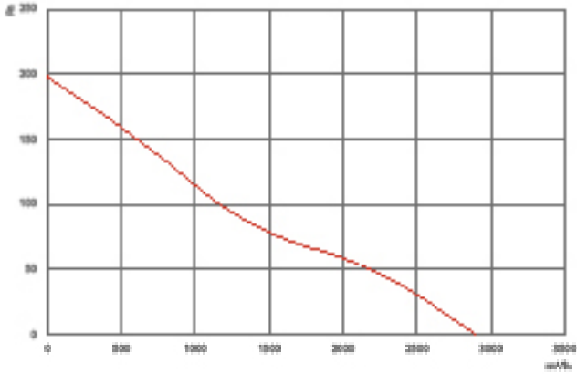
NFDAX/BX 400-5-25
