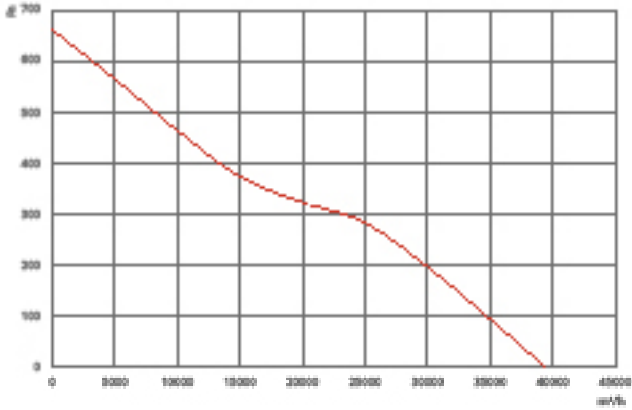
NFDAX/BX 900-5-35
