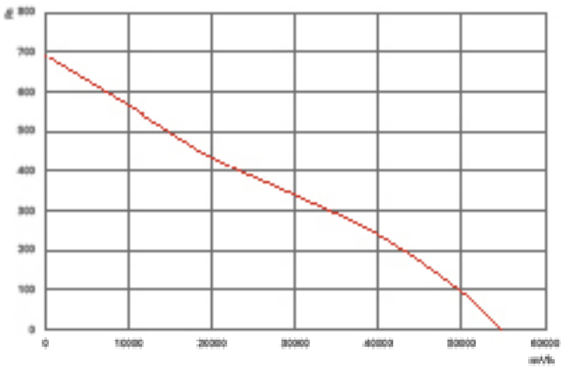
NFDAX/BX 1000-5-40
