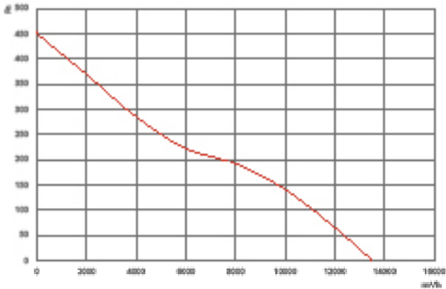
NFDAX/BX 630-5-30
