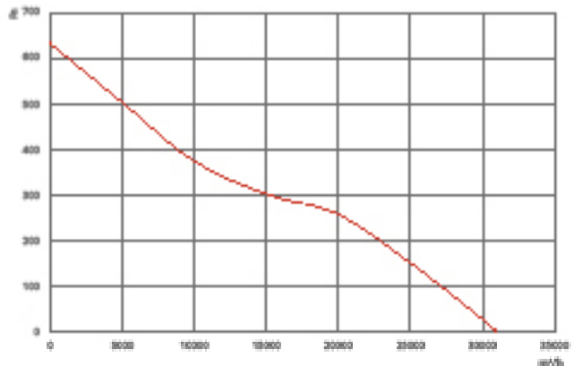
NFDAX/BX 800-5-35
